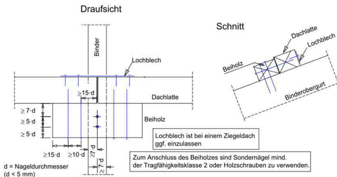
Bild 6: Stoß der Dachlatten mit einem Beiholz und einem Lochblech mit Angabe der Mindestabstände der Latten (dargestellt sind die Mindestnagelanzahlen)
