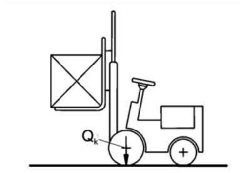
Gabelstapler nach DIN EN 1991-1-1:2010-12 Abschnitt 6.3.2.3
