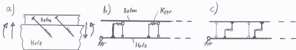
Abb. 2: Beispiel für eine Diskretisierung (globales Stabwerksmodell), auch Modell nach Rautenstrauch genannt
