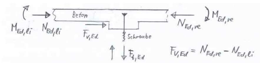
Abb. 6: Schnittgrößen: äußere Kräfte an der Betonknagge
