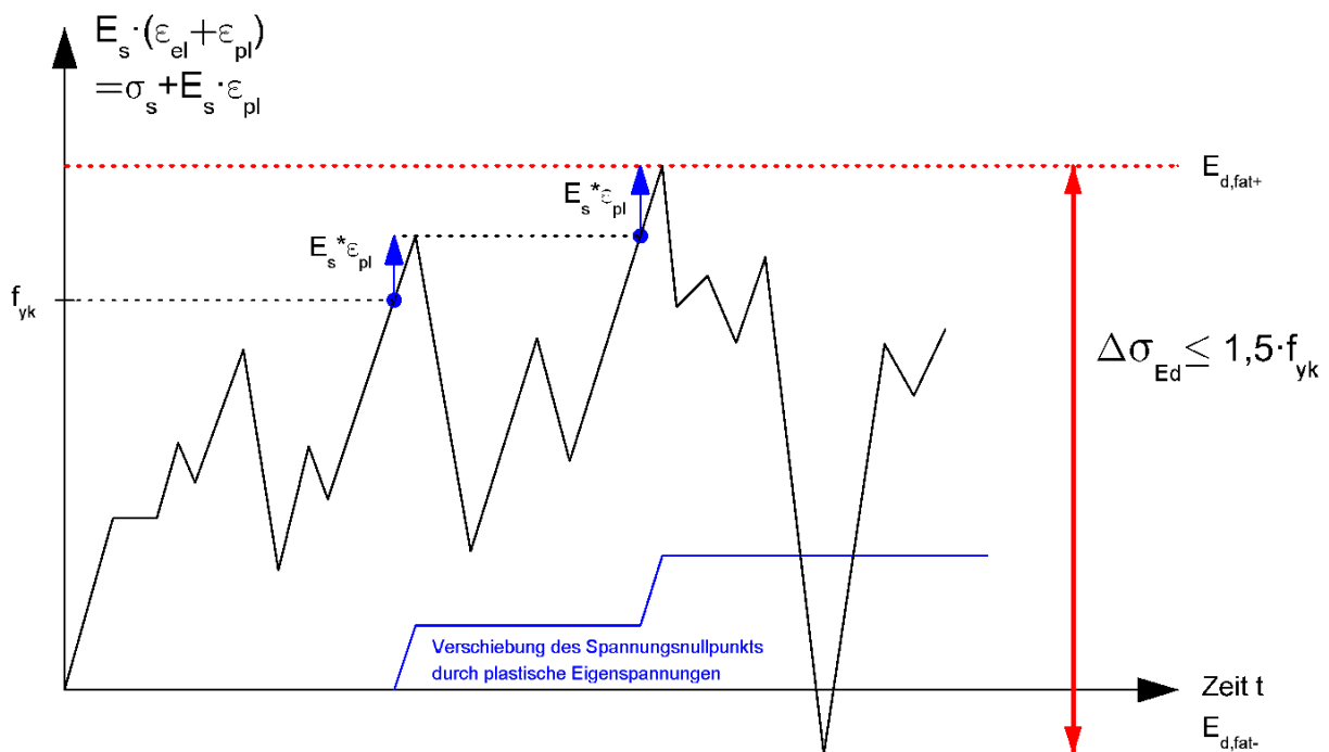
Abb. 1: Beispiel einer Bauteilbeanspruchung mit zeitlich veränderlichen Lasten
