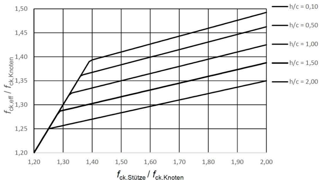
Bild 2 Effektive Betondruckfestigkeit f_{c,eff} nach /1/
