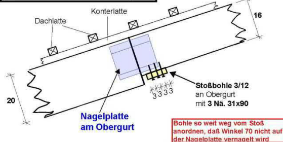
Fig. 4 Durchlaufende Stoßbohle zur Obergurt-Drehsicherung unterseitig des Binders
