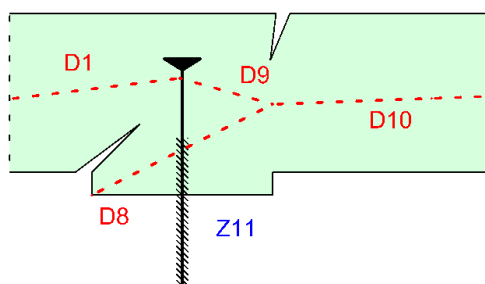
Abb. 7: Bsp. für ein lokales Stabwerksmodell an der 2. Kerve bei mittlerer Schraubenanordnung
