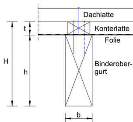
Bild 2: Dachlatte über die Konterlatte auf dem Binderobergurt befestigt Bedingung H/b \leq 4 , hier H = \text{Gurthöhe } h + \text{Höhe der Konterlatte } t
