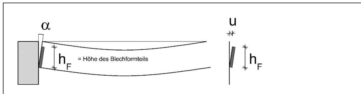
Bild 2: Abschätzung der Verformung
