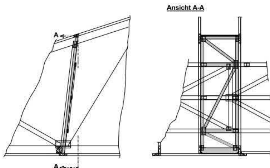
Fig. 3 Anordnung von K-Böcken (K-Verband gem. Fig. 1) zwischen zwei Hauptbindern (Beispiel)
