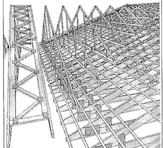
Beispiel 3D-Bild Einschiebung
