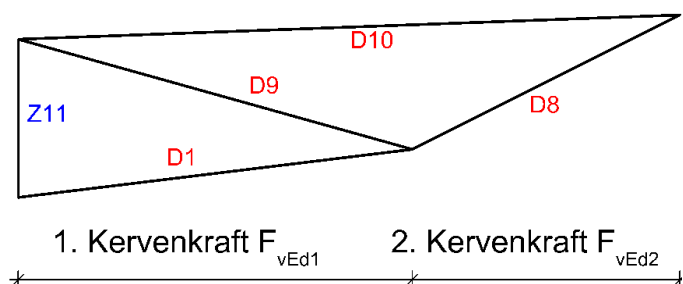
Abb. 7: Bsp. für ein lokales Stabwerksmodell an der 2. Kerve bei mittlerer Schraubenanordnung
