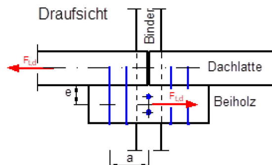
Bild 5b: Definition der Abstände a und e sowie der Kräfte beim tragenden Stoß einer Dachlatte
