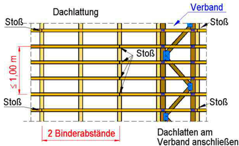
Bild 3: Mögliche Anordnung der Stöße der Dachlatten; Anschluss der Latten an den Verband
