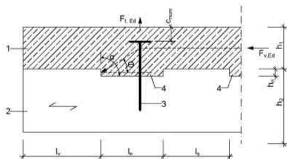
Abb. 1: Bezeichnungen nach Bild 10.2 der DIN CEN/TS 19103 und Kervenbreite b_m
