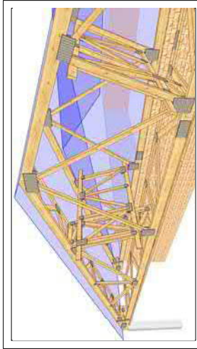
Befestigung des Längsaussteifungssystems am Hauptbau entfällt
