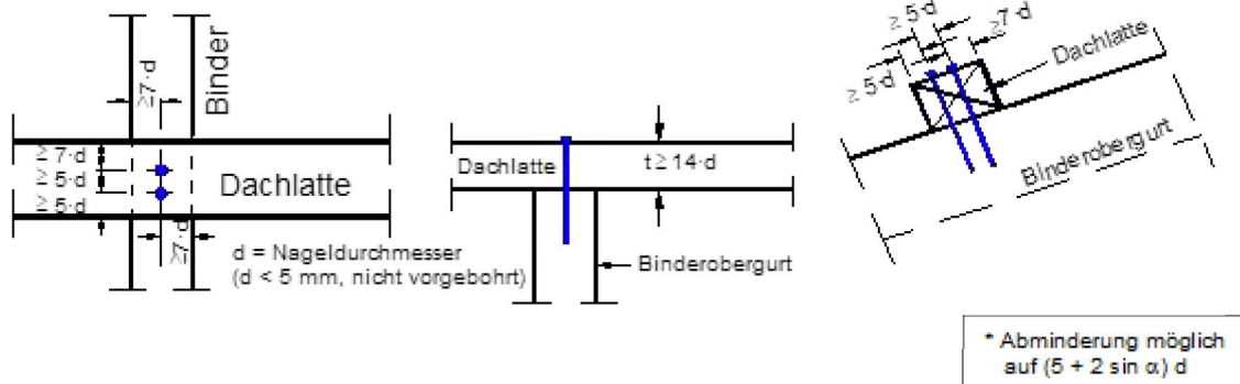
Bild 4a: Befestigung durchlaufender Dachlatten aus Fichte/Tanne mit einer Dicke t \geq 14 \cdot d und für Kiefer mit einer Dicke t \geq 7 \cdot d ; Mindestabstände für nicht vorgebohrte Nägel d < 5 mm
