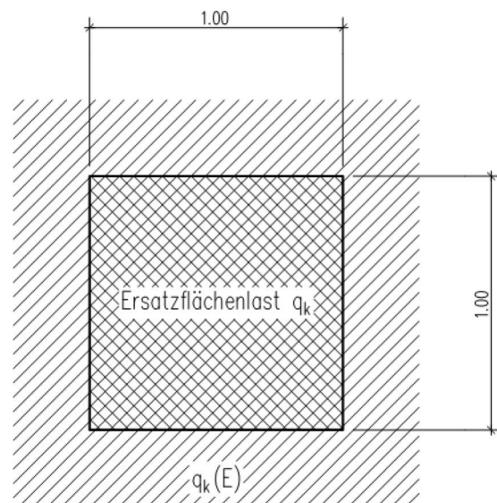
b) Lastansatz mit Ersatzflächenlast
