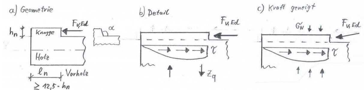
Abb. 8: Kräfte an der Holzknaagge
