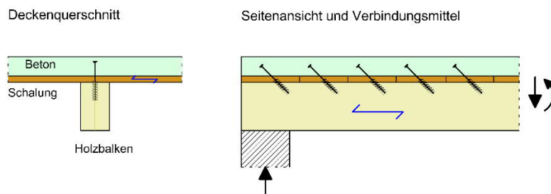
Abb. 3: HBV-Decke mit Zwischenschicht
