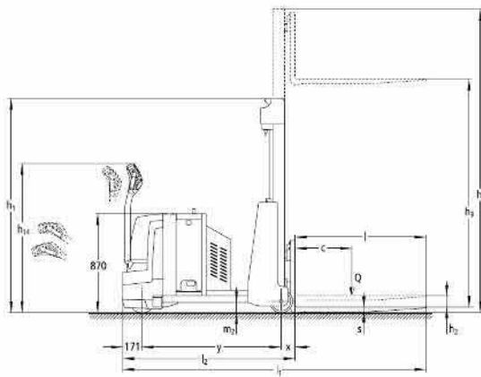
Handgeführtes Transportfahrzeug
