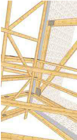
3D-Ansicht
