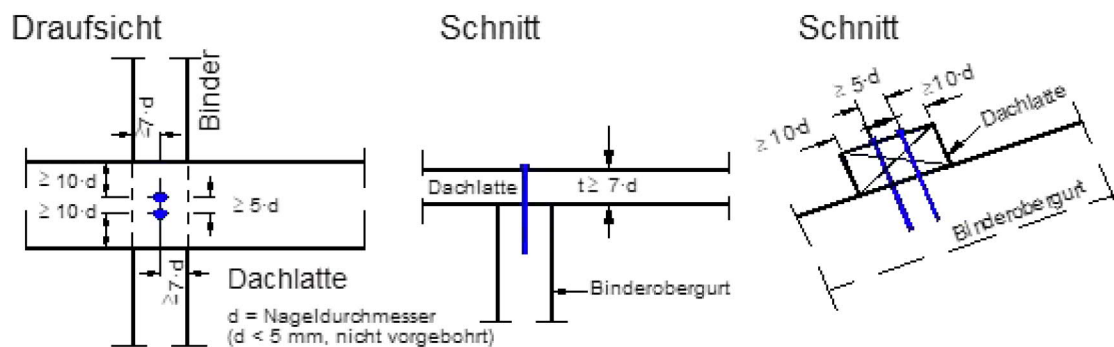
Bild 4b: Befestigung durchlaufender Dachlatten aus Fichte/Tanne mit einer Dicke t \geq 7 \cdot d Mindestabstände für nicht vorgebohrte Nägel d < 5 \text{ mm}
