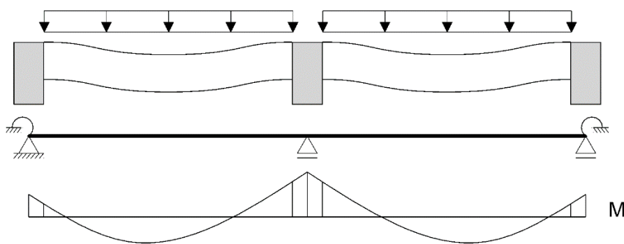
Bild 3: Beispiele für die Anwendung in unterschiedlichen statischen Systemen die Verformung ist zur Verdeutlichung überhöht dargestellt
