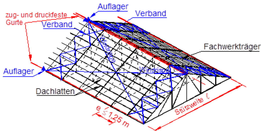
Bild 1: Fachwerkträger mit der Stützweite l , den Verbänden in der Dachebene, den druck- und zugfesten Gurten an Traufe und First und der Abspannung durch Windrispen
