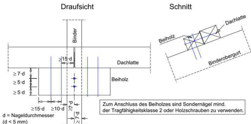
Bild 5a: Tragender Stoß einer Dachlatte mit einem Beiholz; Mindestabstände für nicht vorgebohrte Nägel d < 5 \text{ mm} (dargestellt sind die Mindestnagelanzahlen)
