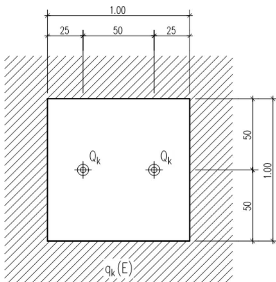
a) Lastansatz mit Radlasten
