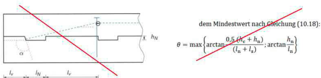
Abb. 4: Unvollständiges Stabwerksmodell; Bild aus [5] und Gl. (10.18) aus DIN CEN/TS 19103 [1]
